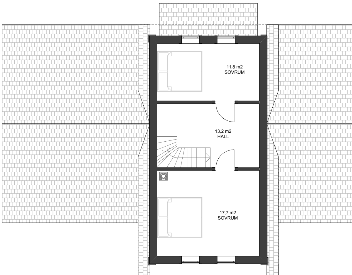
PLAN 2 1:100
