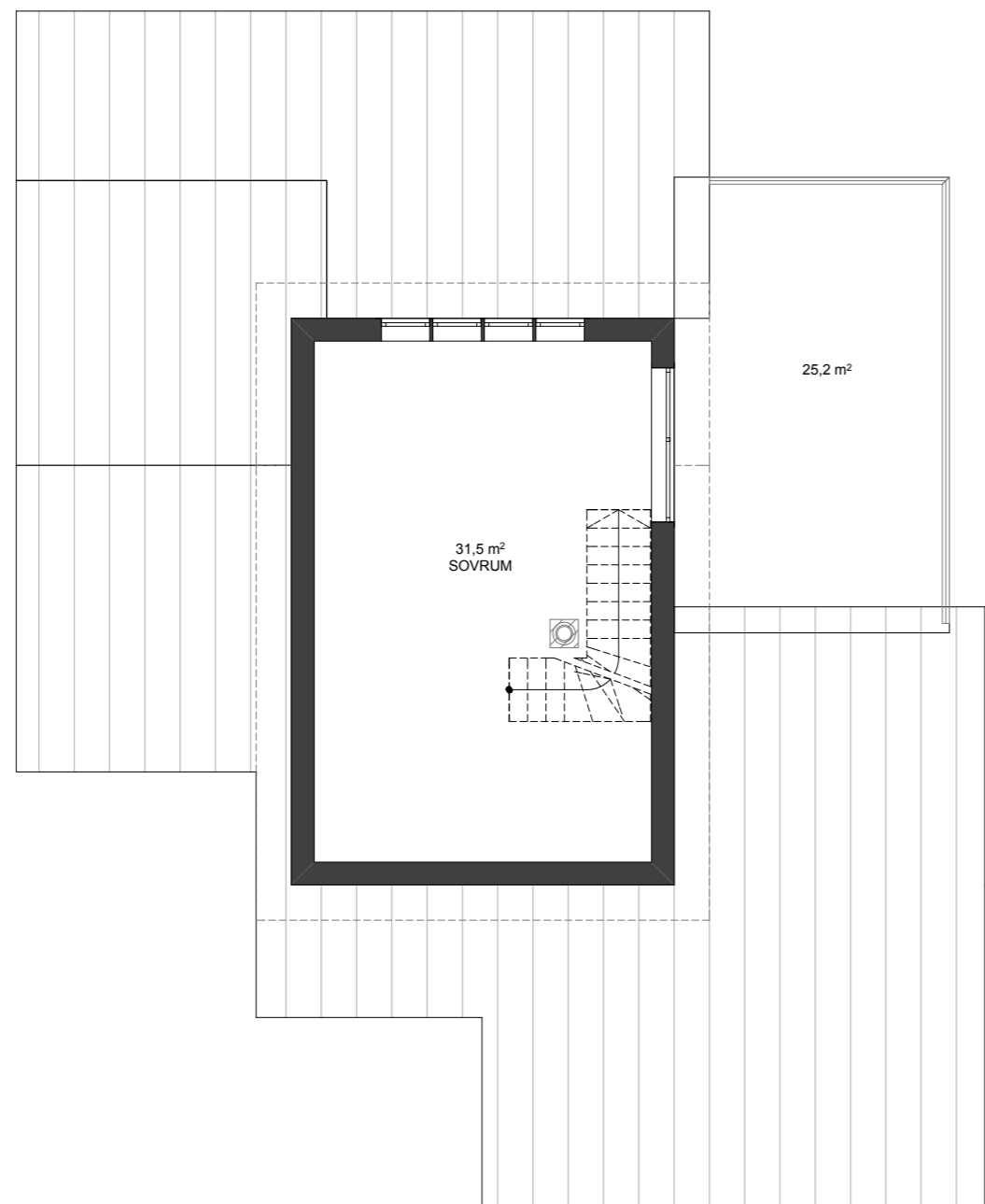
PLAN 2 1:100
