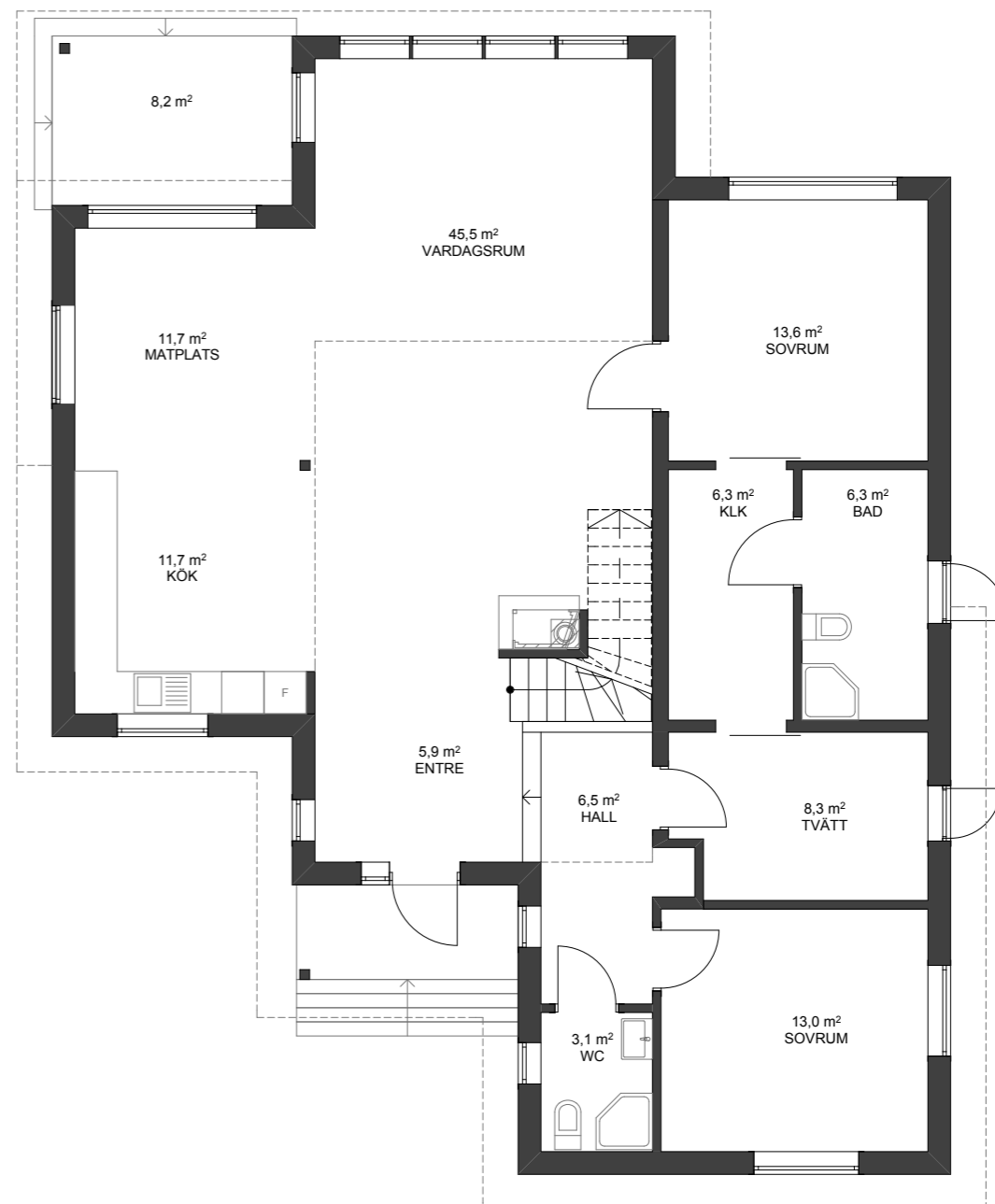
PLAN 1 1:100
