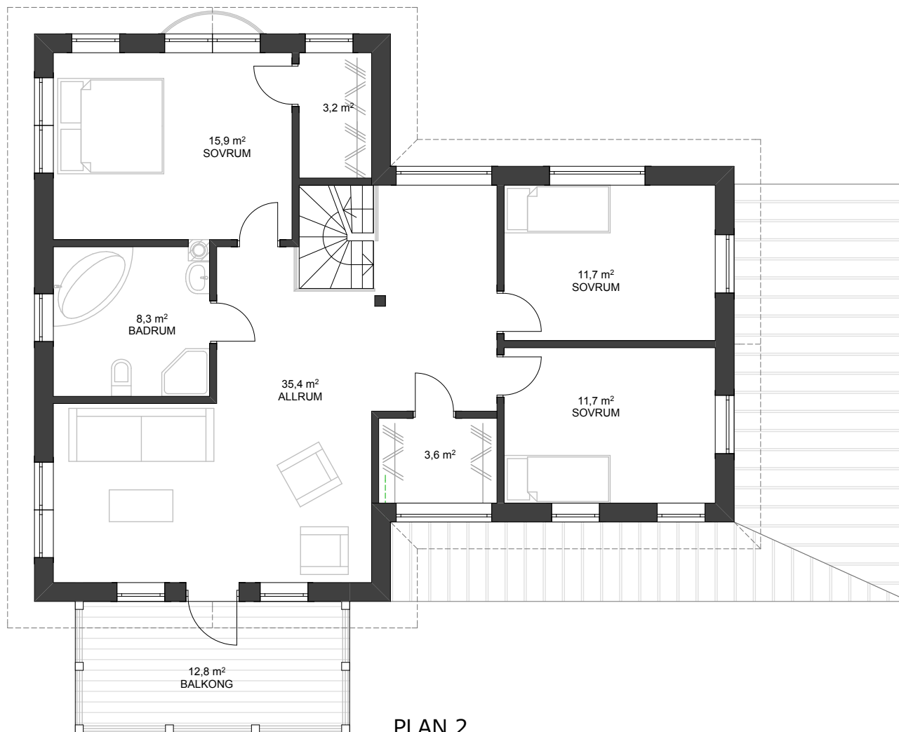
PLAN 2 1:100
