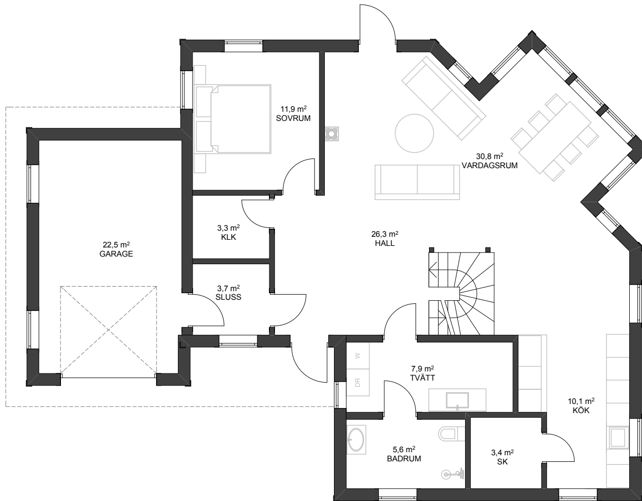
PLAN 1 1:100
